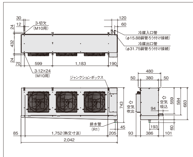
US-T10H1 / US-T10MH1 / US-T10LH1 (単位:mm)
