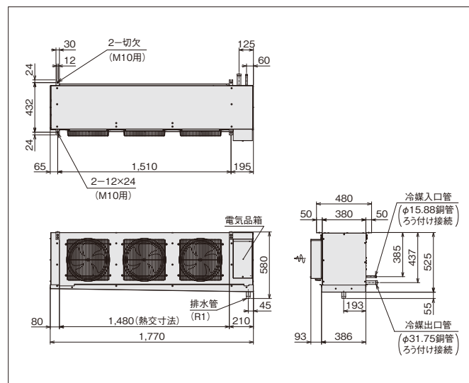
US-T6H / US-T6MH / US-T6LH (単位:mm)
