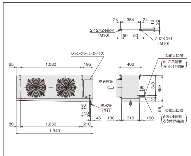
US-T4H1 / US-T4MH1 / US-T4LH1 (単位:mm)
