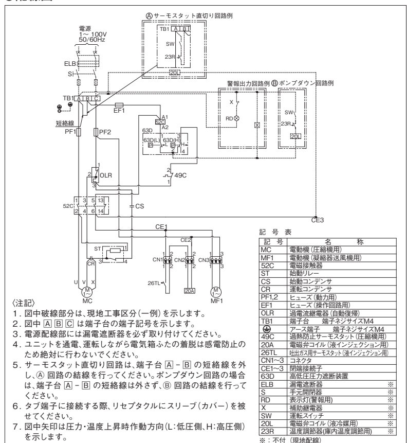
●配線図
