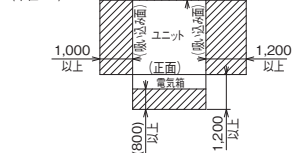
サービススペース (単位:mm)
