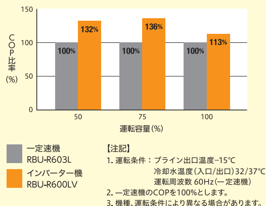
●COP比較(一定速機60馬力・インバーター機60馬力の場合)
