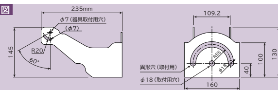
壁直付用アーム RBMEV010
