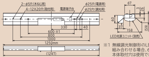
寸法図
