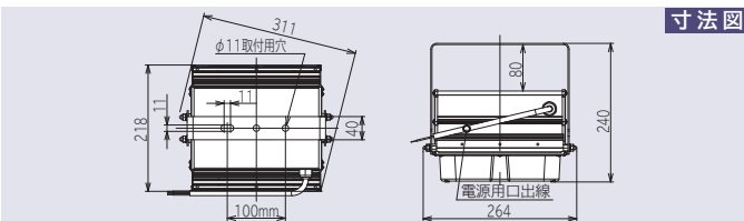
寸法図
