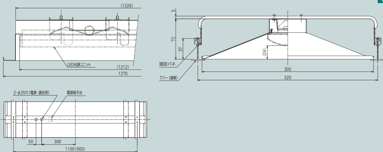
寸法図
