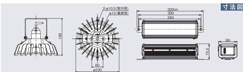
寸法図
