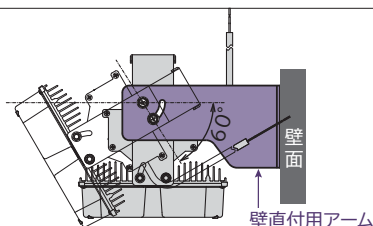
壁直付用アーム
