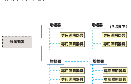
結線図(共通)
