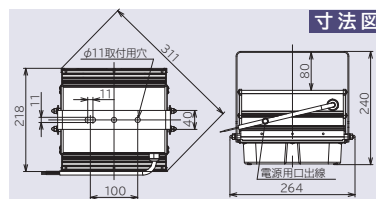
寸法図
