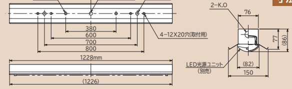
寸法図
