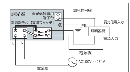
〈結線図〉 1ヶ所点滅:下図の通り結線してください。
