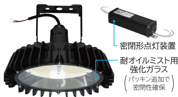
高天井用LEDランプ アームタイプ 防湿・防雨形(オイルミスト・粉じん対応)
