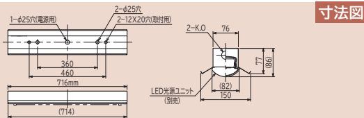
寸法図
