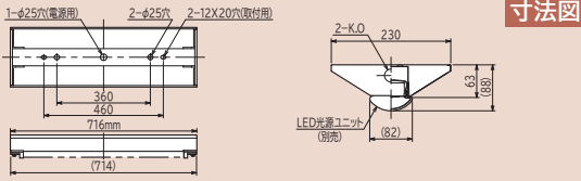
寸法図
