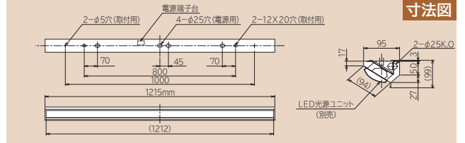
寸法図
