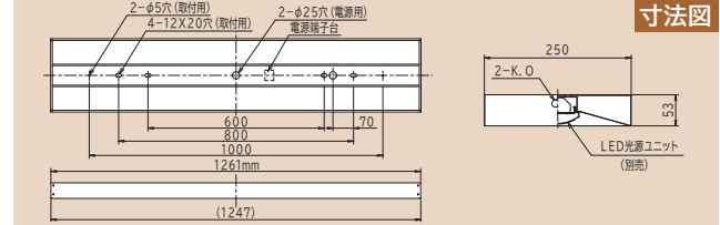
寸法図
