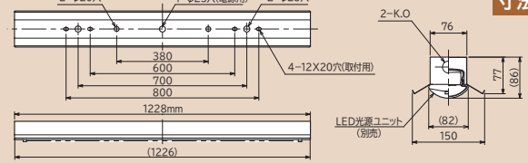
寸法図
