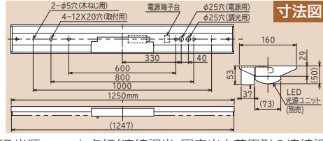
逆富士形 幅160mm 品名コード 在庫区分 価格(税別)☆ ZNC4A2 6253-3718 ○ 49,000円
