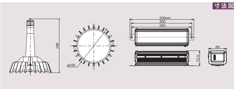
寸法図
