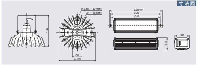
寸法図
