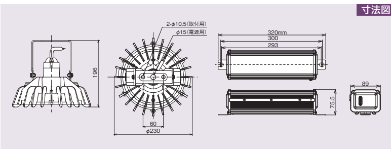
寸法図
