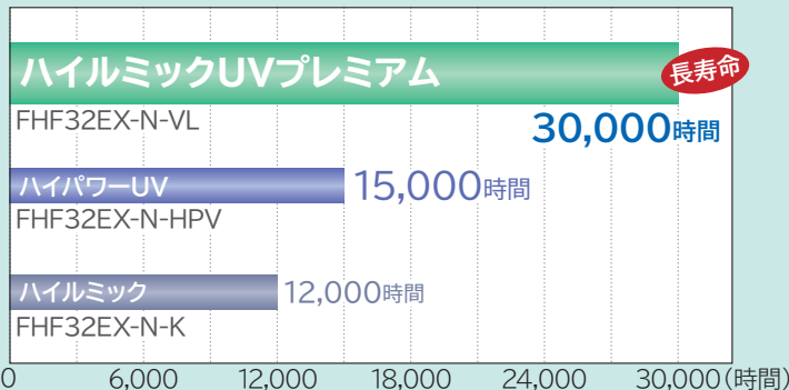
【高周波点灯専用形(Hf)蛍光ランプの定格寿命比較】
