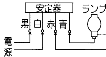
結線図
