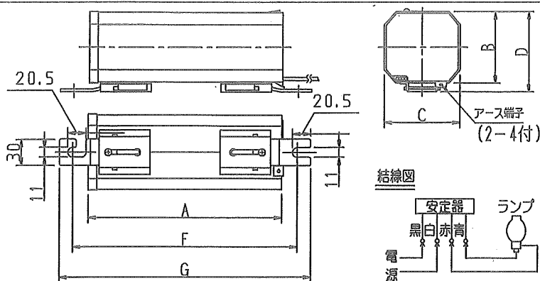
寸法表
