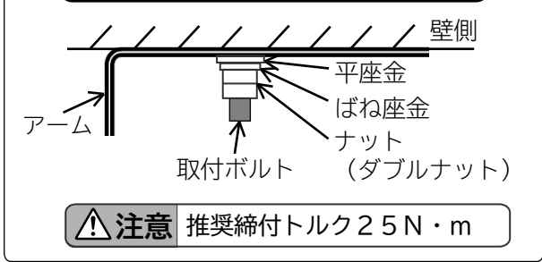
図2 器具取付
