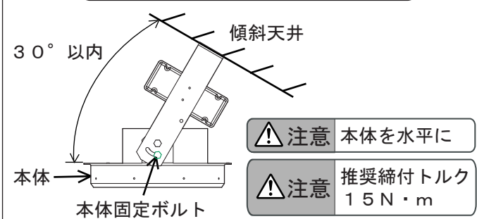
図3 傾斜天井に取り付ける場合
