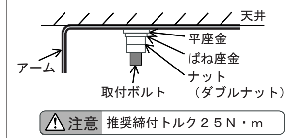
図2 器具取付
