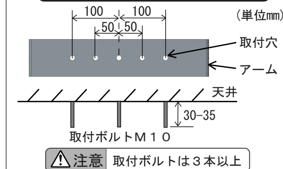
図1 取付ボルト施工寸法
