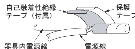
電源線の接続(図4)
