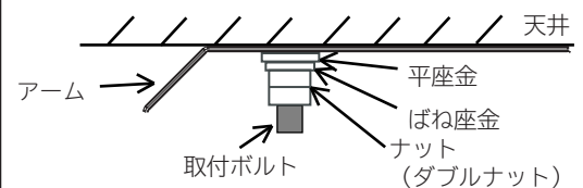
図2 器具取付
