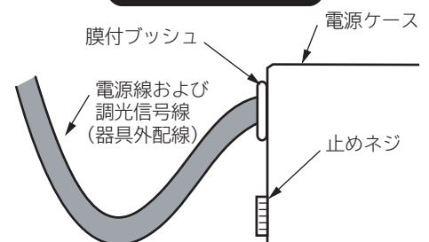
図5 配線の配置
