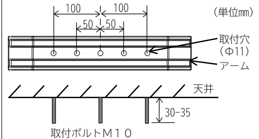
図1 取付ボルト施工寸法
