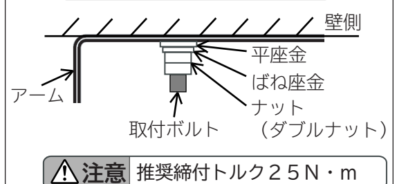
図3 角度を変更する場合
