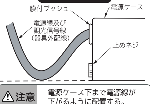
図5 配線の配置
