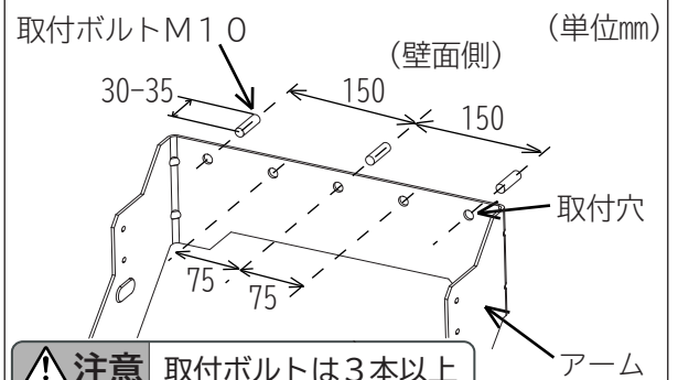
図2 器具取付
