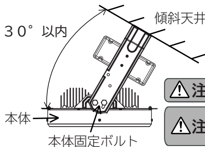
図3 傾斜天井に取り付ける場合
