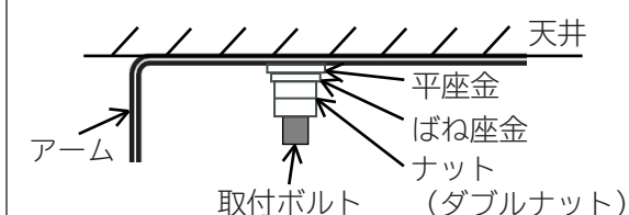
図2 器具取付
