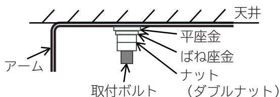
図2 器具取付
