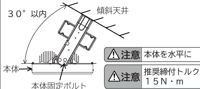
図3 傾斜天井に取り付ける場合
