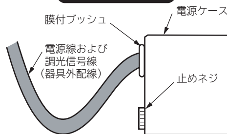
図5 配線の配置
