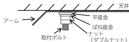
図2 器具取付
