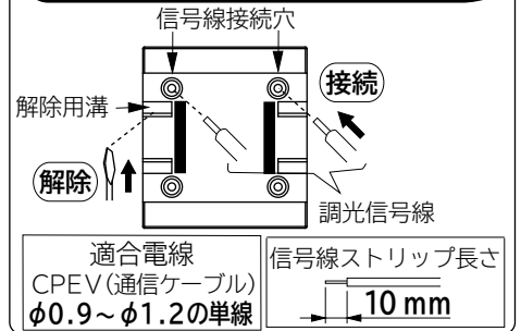
図6 調光端子台の接続と解除
