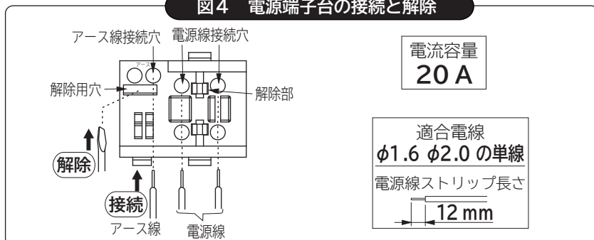
図4 電源端子台の接続と解除
