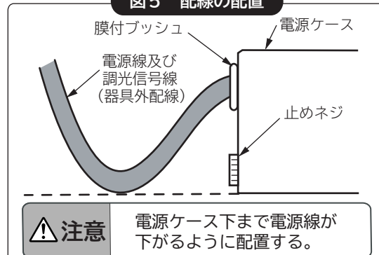
図5 配線の配置
