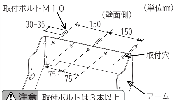
図2 器具取付
