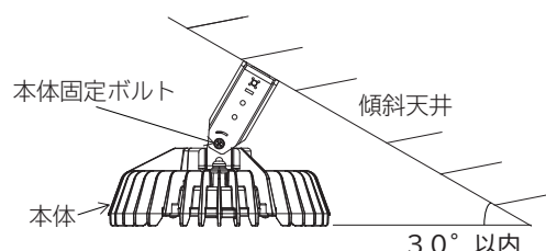
図5 傾斜天井に取り付ける場合
