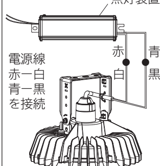
図4 配線接続
