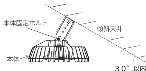
図5 傾斜天井に取り付ける場合
