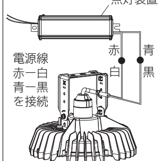
図4 配線接続
