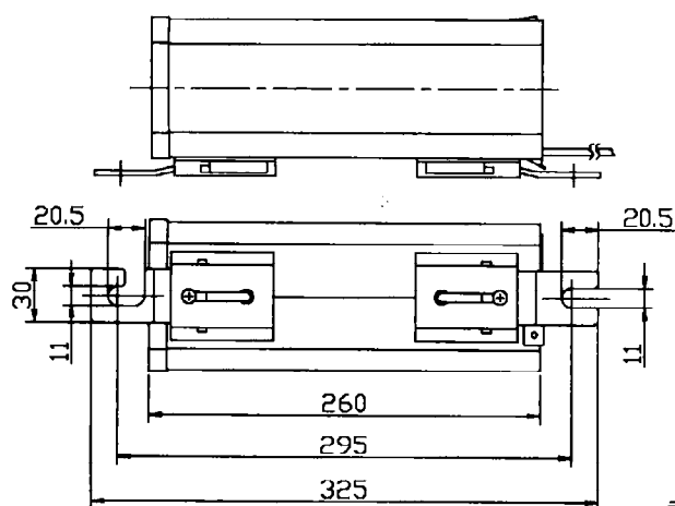
寸法表
