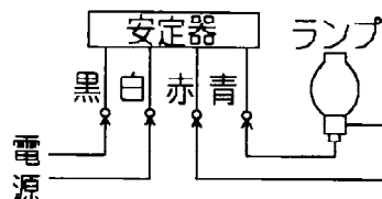
結線図
