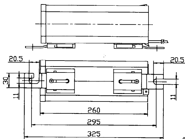
寸法表
