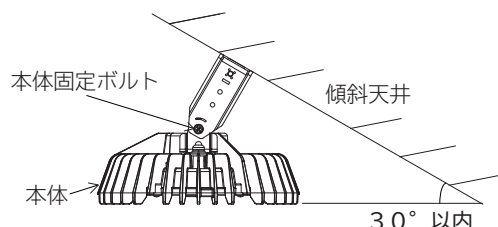
図5 傾斜天井に取り付ける場合
