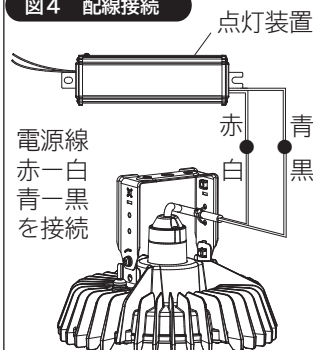
図4 配線接続
