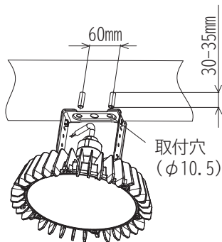
図1 取付ボルト施工寸法
