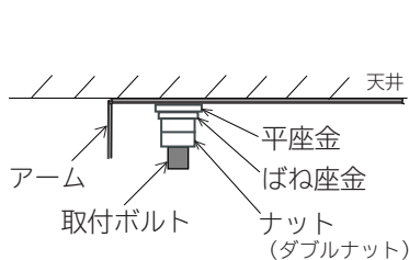
図2 LEDランプの取り付け
