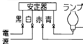
結線図
