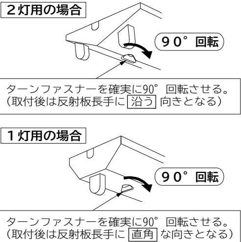
反射板の取り付けかた (図4)
