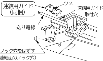
電源端子台の接続と解除 (図3)
