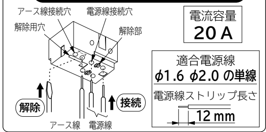
調光端子台の接続と解除 (図3)
