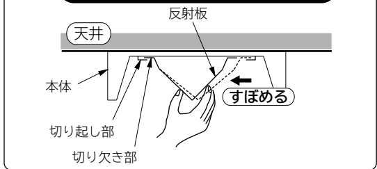
反射板の取り付けかた (図4)
