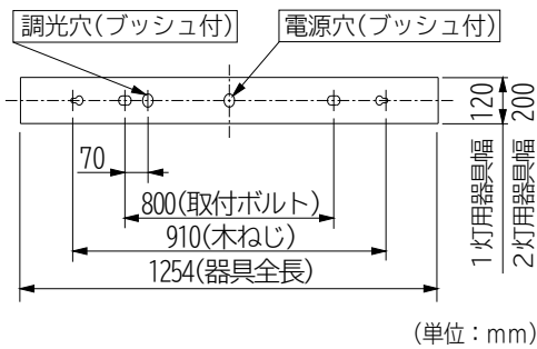
連結のしかた (図2)
