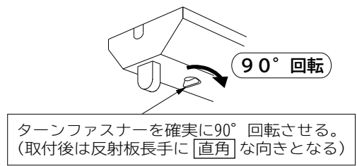
ランプの取り付けかた (図6)
