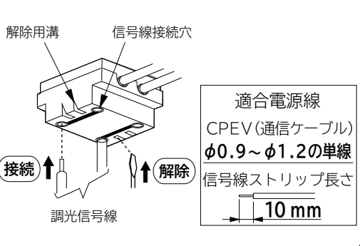
調光端子台の接続と解除 (図4)
