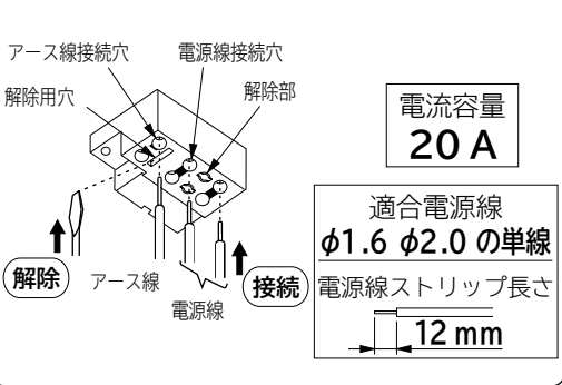
電源端子台の接続と解除 (図3)
