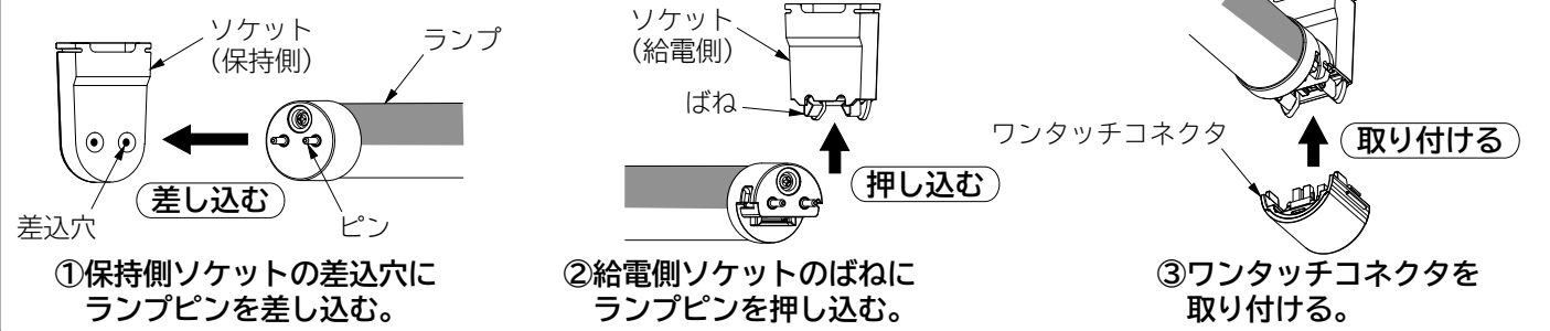
ランプの取り付けかた (図6)
