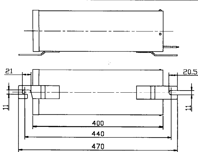
寸法表
