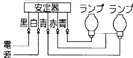
結線図
