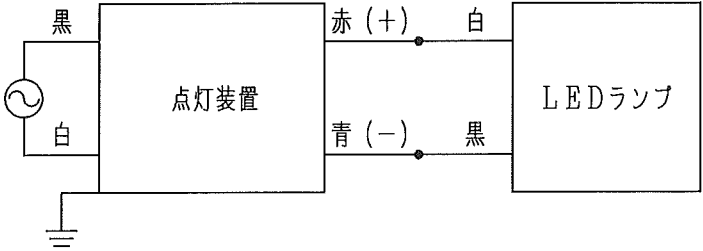
〔結線図〕
