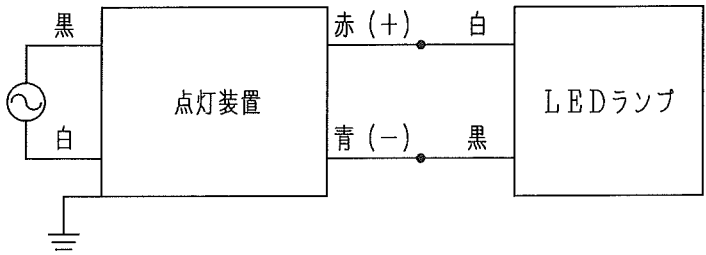
〔結線図〕
