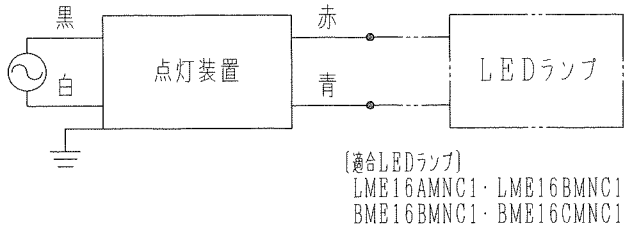
〔結線図〕
