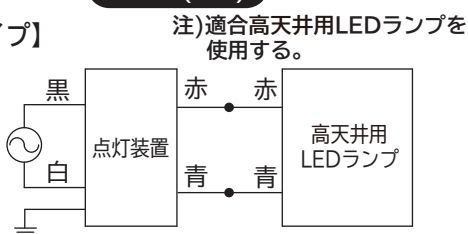
配線図(図3)
