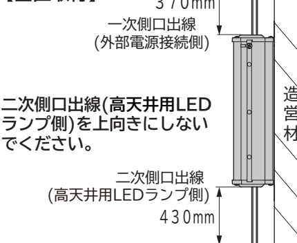
取付方向(図1)
