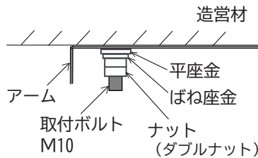
図2 LEDランプの取り付け
