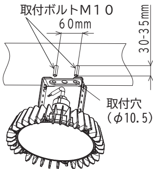
図1 取付ボルト施工寸法
