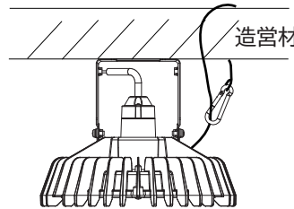
図3 落下防止ワイヤーの取り付け
