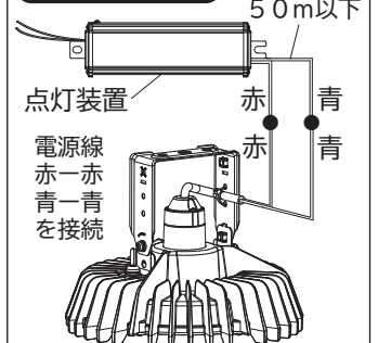
図4 配線接続
