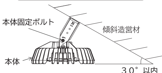
図5 傾斜造営材に取り付ける場合
