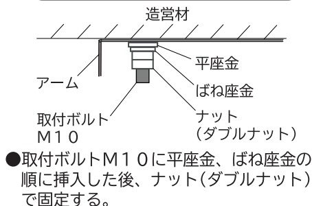
図2 LEDランプの取り付け
