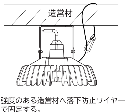
落下防止ワイヤーの取り付け(図3)
