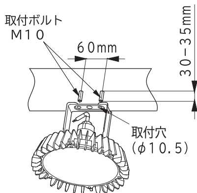
取付ボルト施工寸法(図1)
