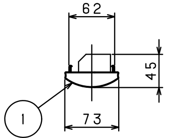
右側面図（S=1/5）
