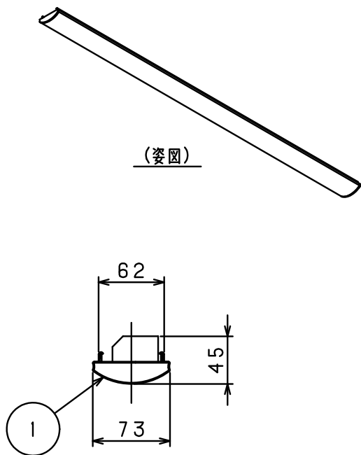
右側面図（S=1/5）
