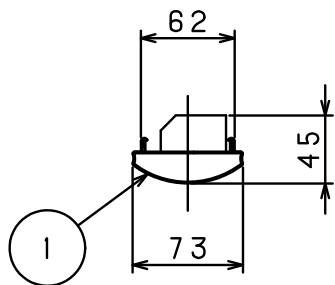
右側面図（S=1/5）
