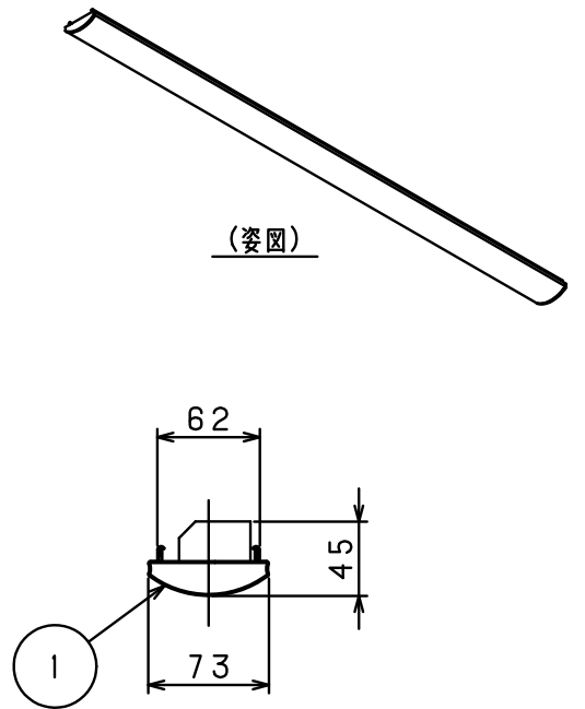
右側面図（S=1/5）
