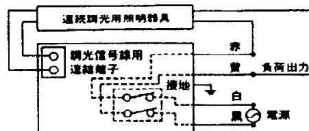
配線図(200V用) 1カ所点滅(2カ所点滅は出来ません。)
