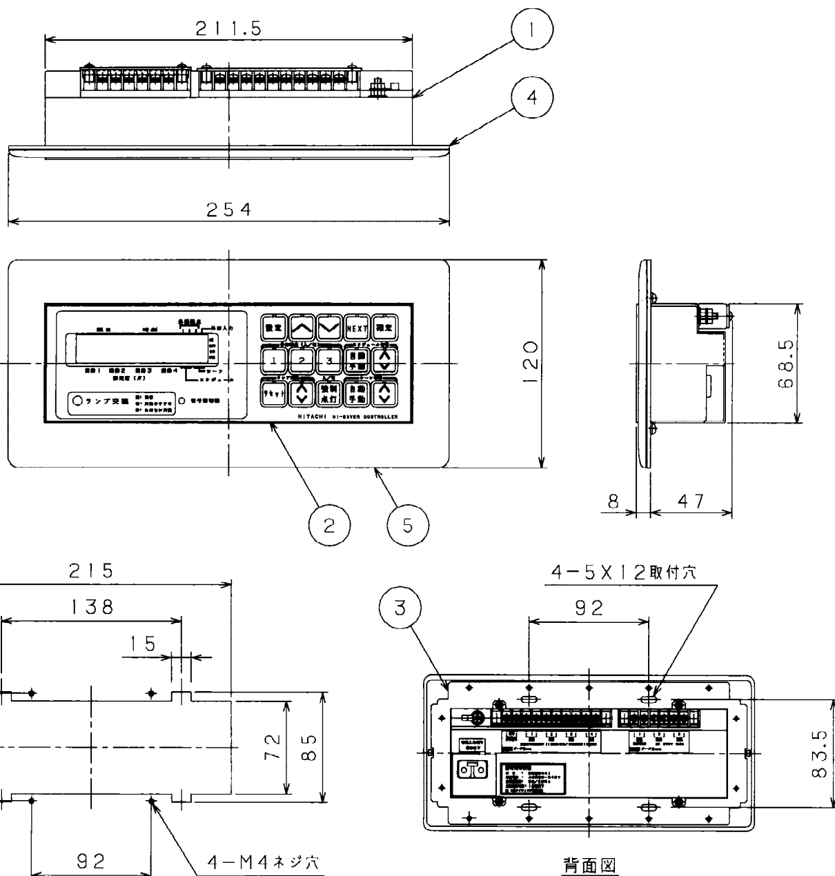
取付加工図（盤取付の場合）
