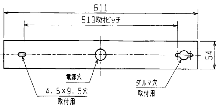
取付寸法図
