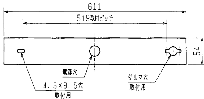
取付寸法図
