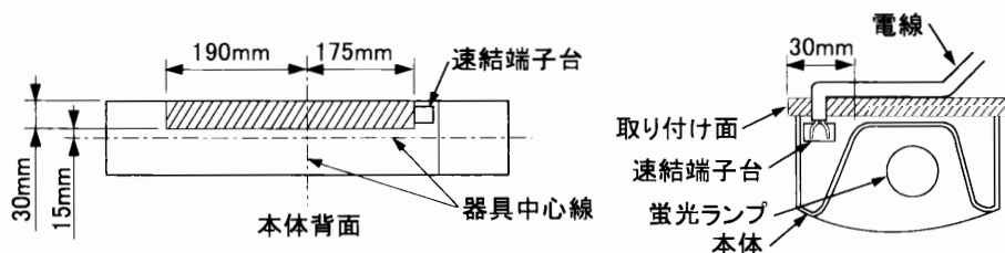
●器具の取付け面の電線配線施工範囲
