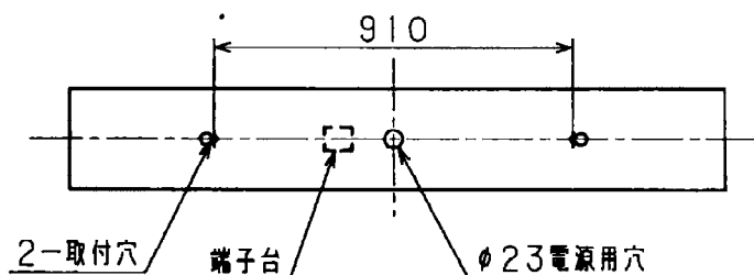
取付寸法図
